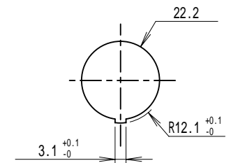
パネル穴明寸法
