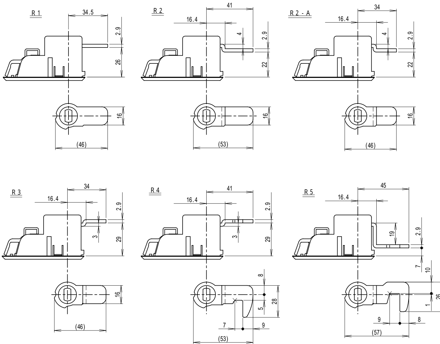
* ベロカン詳細図
