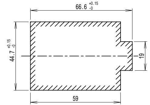
パネル穴明寸法
