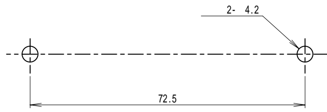
取付穴寸法
